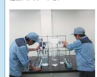
事業場排水処理実験装置
